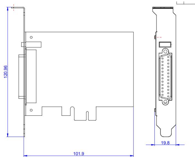
PCIE 主卡
