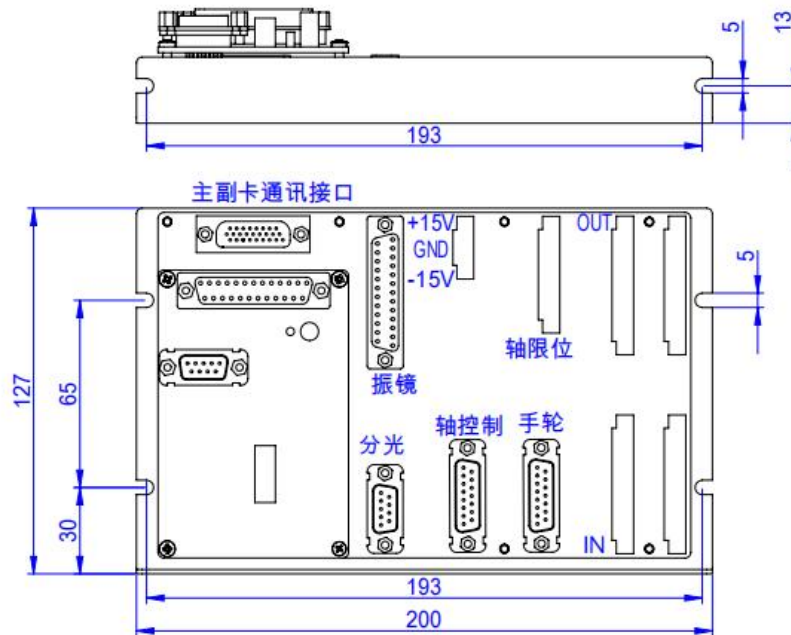
PCIE 端子板
